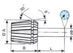
C01 ER Spring Collet Chuck System
